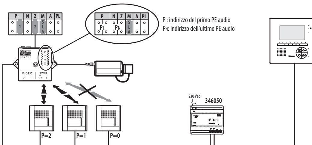
Abbinamento accensione telecamera solo ad alcuni PE audio presenti nell'impianto (max. 5)
