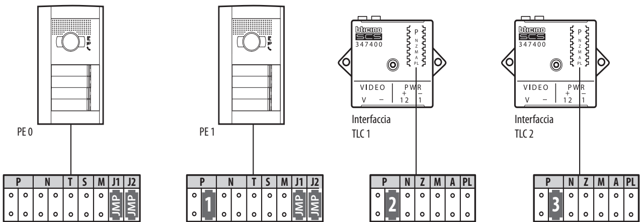
Impianto con 2 PE video e 2 telecamere.
