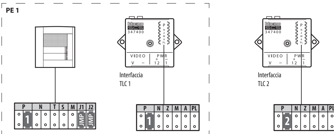
Impianto con PE audio e 2 telecamere (TLC 1 associata al PE)
